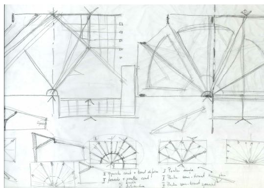
Croquis charpente
