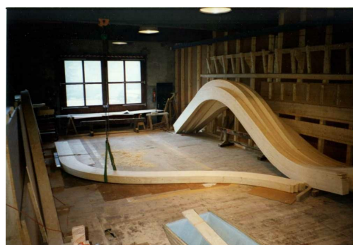
Cintrage des poutres en atelier
